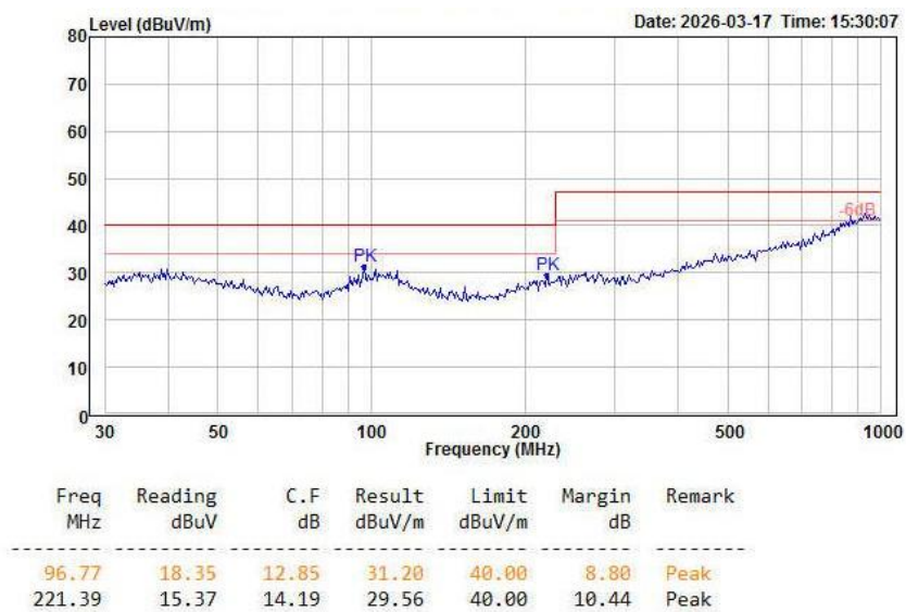
图 6-7 辐射测试水平方向
