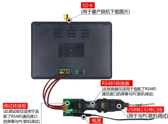
图 1-5 RS485 调试工具图
