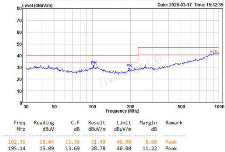
图 6-8 辐射测试垂直方向
