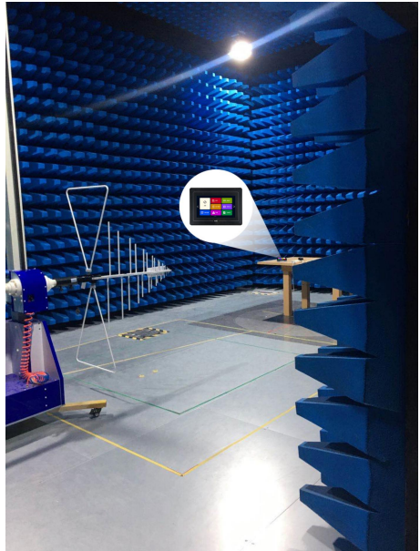
图 6-6 辐射测试图
